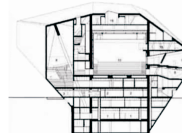
Presjek sjever – jug
