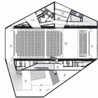
Tlocrt zgrade s velikom dvoranom
