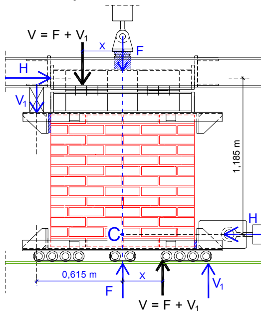
Slika 9. Sile koje djeluju na uzorak tijekom ispitivanja i ovisnost vertikalne sile V_1 o horizontalnoj sili H
