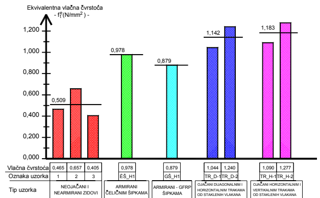
Slika 14. Ekvivalentne vlačne čvrstoće зида i njihove prosječne vrijednosti
