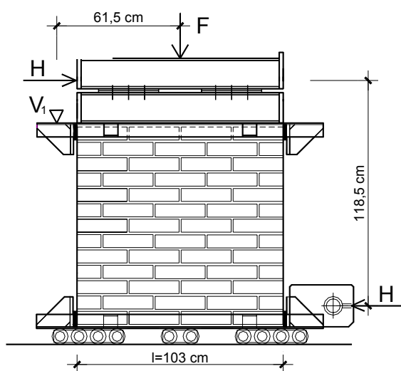
Slika 5. Skica uzorka i adaptera tj. opreme za ispitivanje na stalno vertikalno i promjenjivo horizontalno opterećenje. H: horizontalna promjenjiva sila; F: vertikalna sila; V 1 : vertikalno pridrzanje koje ne dopušta odizanje lijevog ruba zida
