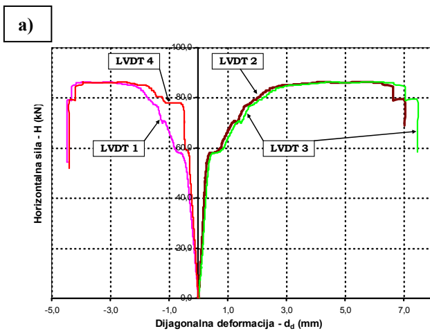
Slika 13. Prikaz odnosa „Sila – dijagonalna deformacija (LVDT br. 1 i 4 u smjeru tlačne a LVDT 2 i 3 u smjeru vlačne dijagonale)“, a) za nearmirani zid (lijevo) i b) za zid ojačan dijagonalnim i horizontalnim trakama od staklenih vlakana
