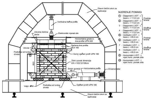
Slika 8. Shema uređaja za ispitivanje i uzorka
