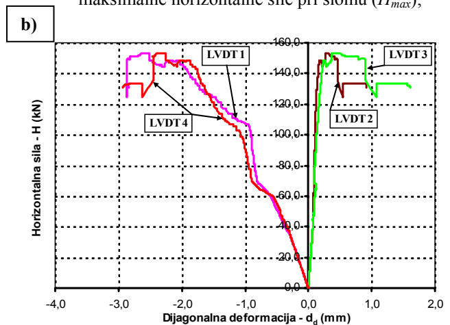
Slika 13. Prikaz odnosa „Sila – dijagonalna deformacija (LVDT br. 1 i 4 u smjeru tlačne a LVDT 2 i 3 u smjeru vlačne dijagonale)“, a) za nearmirani zid (lijevo) i b) za zid ojačan dijagonalnim i horizontalnim trakama od staklenih vlakana
