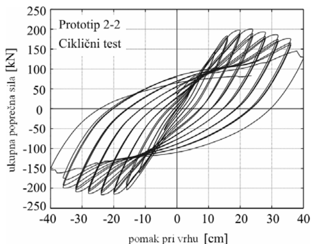
Slika 9. Histerezni odziv pri cikličnom ispitivanju uzorka 2-2 (sila je mjerena za cijelu konstrukciju, sastavljenu od 6 stupova)
