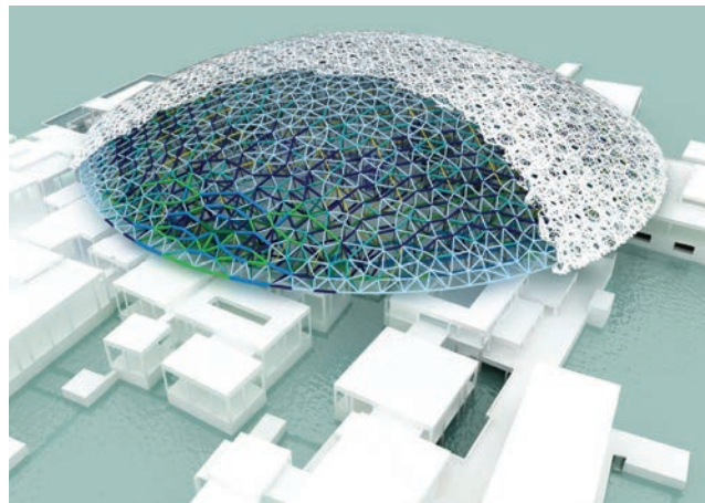
Model rešetkaste kupole
